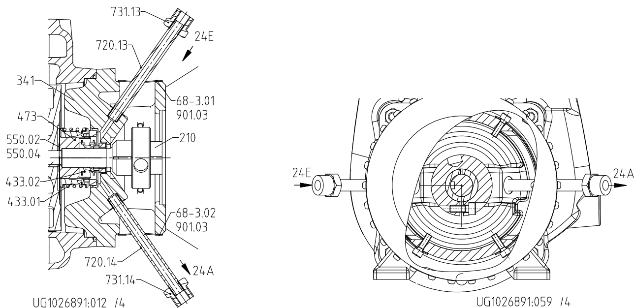
Рис. 12: Исполнение с двойным торцовым уплотнением в тандемном расположении
