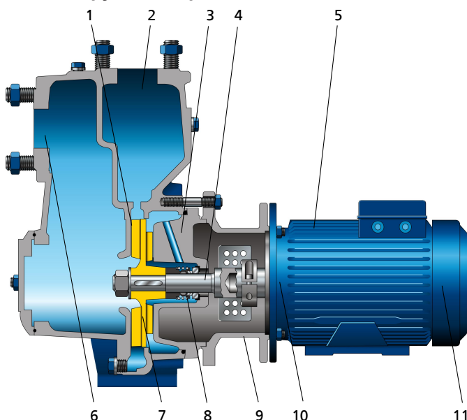
Рис. 3: Сечение
