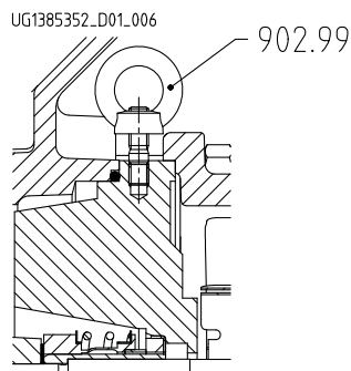
Рис. 8: Вспомогательное средство для монтажа с рым-гайкой
