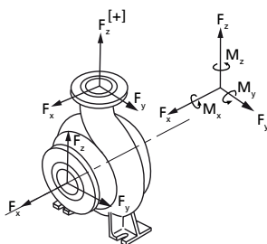
Рис. 5: Силы и моменты, действующие на патрубки насоса
