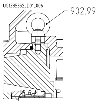
Рис. 6: Вспомогательное средство для демонтажа с рым-гайкой
