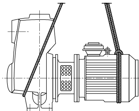
Рис. 1: Транспортировка насосного агрегата
