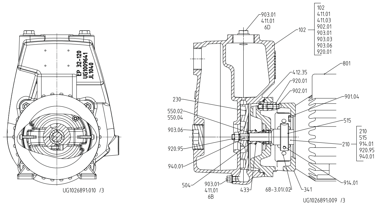
Рис. 11: Исполнение с одинарным торцовым уплотнением
