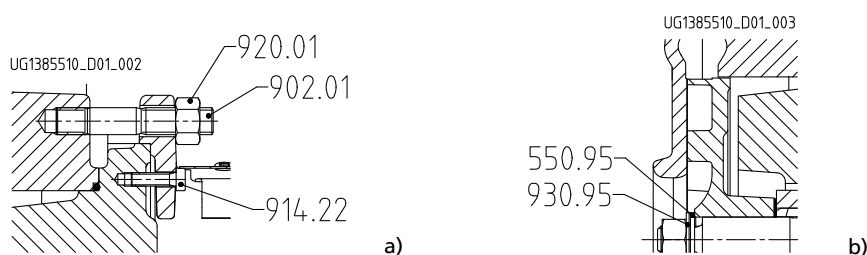
Рис. 14: а) Зажимная крышка корпуса б) Крепление рабочего колеса при узле вала 25
