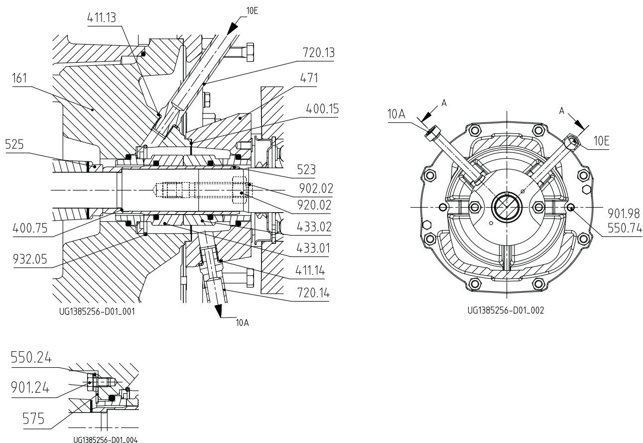
Рис. 16: Исполнение с двойным торцевым уплотнением типа «спина к спине»
