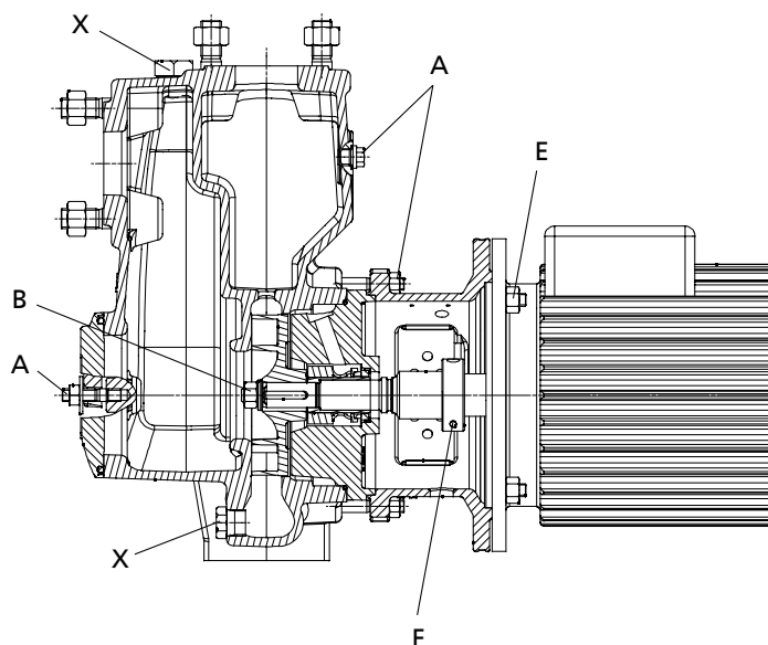
Рис. 10: Места затяжки резьбовых соединений
